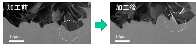
SEMIによる砥粒の観察
