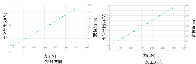
カセンサの検定結果
