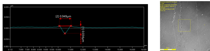
レーザー顕微鏡による加工後のワーク表面形状の観察
