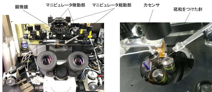
加工実験装置のセットアップ
