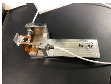
試作したカセンサ
