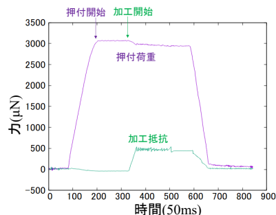
押付荷重と加工反力のグラフ
